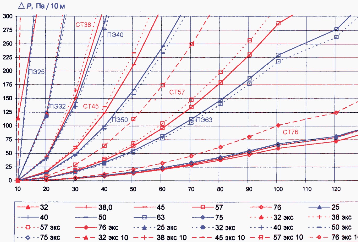
"Удельные потери давления для стальных и полиэтиленовых труб (новых и бывших в эксплуатации) низкого давления"
