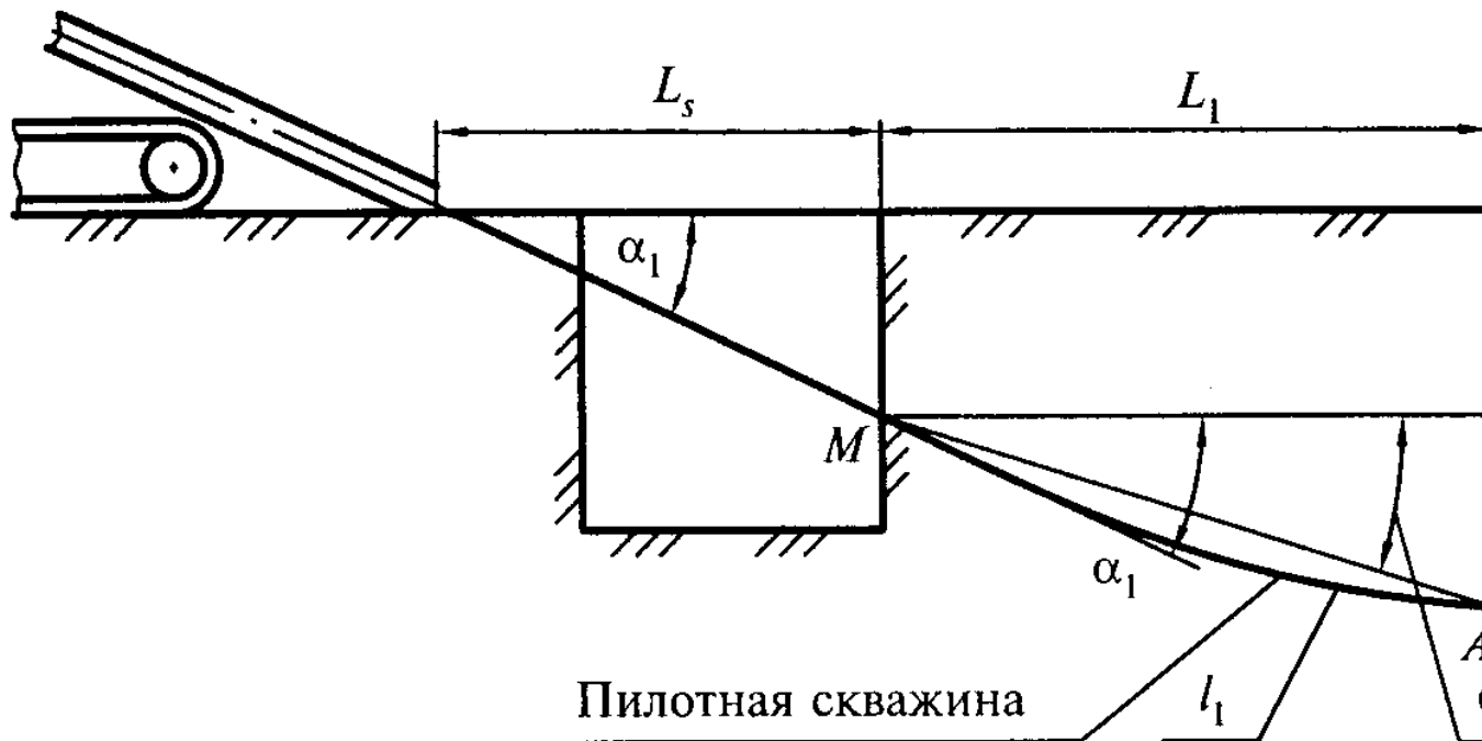
Рисунок Л.2 — Схема забурирования пилотной скважины
