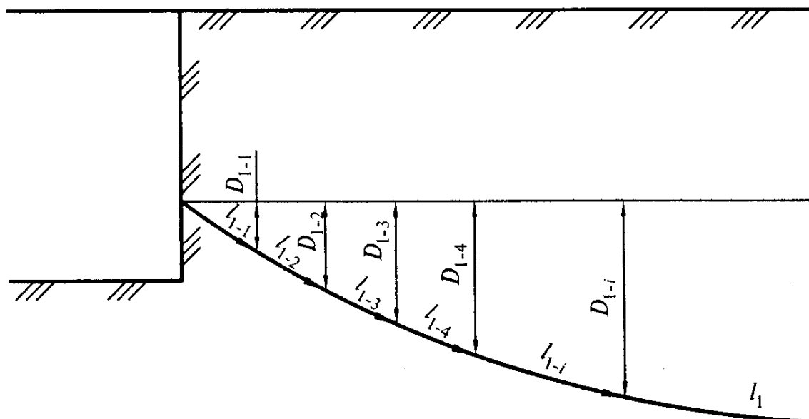
Рисунок Л.3 — Схема перехода пилотной скважины от максимального угла забуривания к нулевому углу
