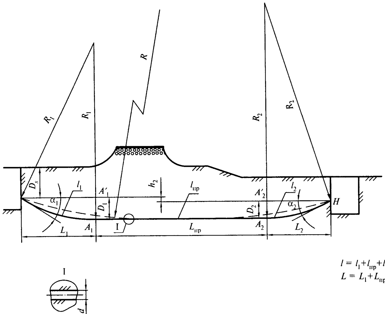
Рисунок Л.1 — Основные геометрические параметры трассы
