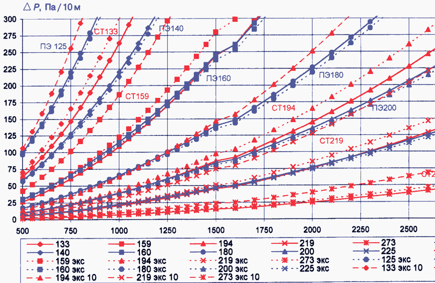
Газопроводы из стальных труб низкого, среднего и высокого давления
